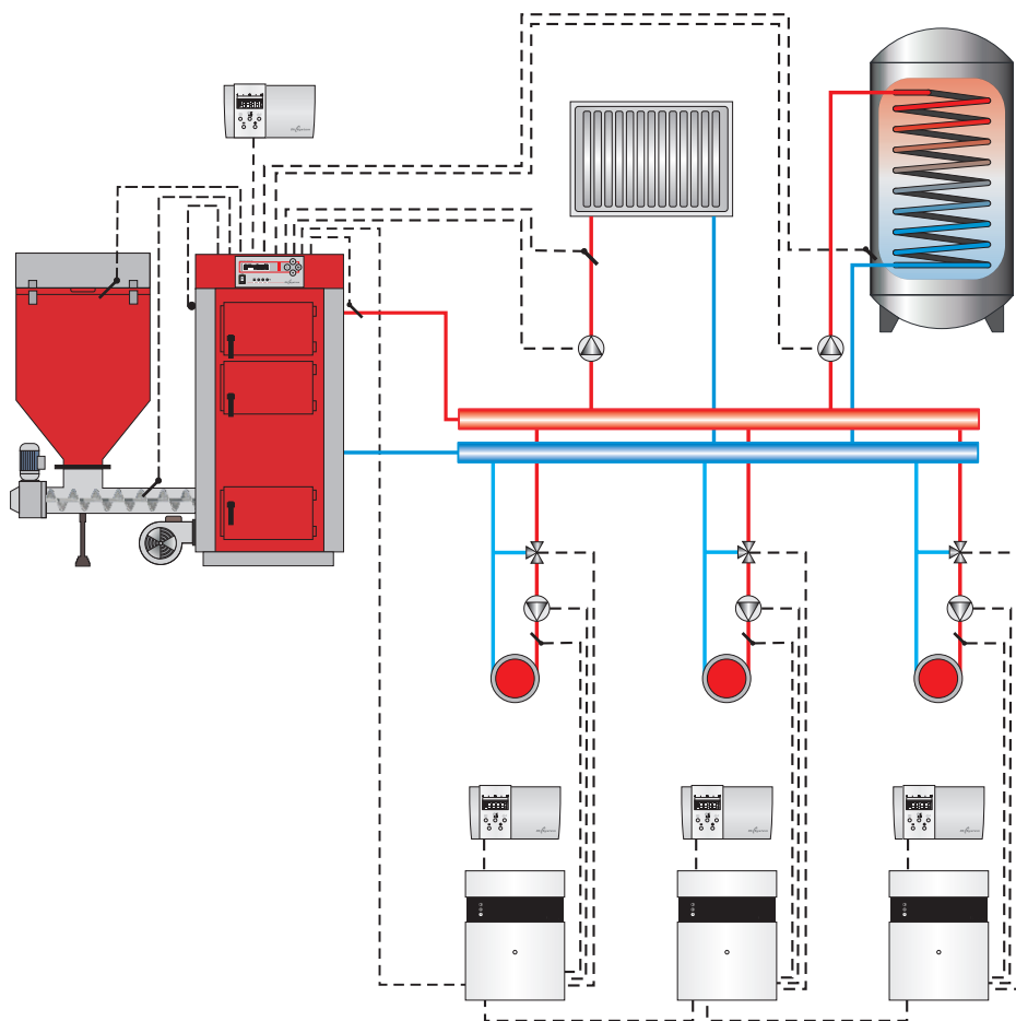
Rys. 5 Przykładowy schemat instalacji z podłączonymi trzema modułami rozszerzającymi DKMZ 1 Obiegu 3, Obiegu 4 i Obiegu 5.
