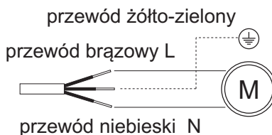
Rys. 4 Schematy podłączenia przewodu zasilającego do dmuchawy i pomp (w zależności od wersji regulatora)
