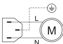
Rys. 4 Schematy podłączenia przewodu zasilającego do dmuchawy i pomp (w zależności od wersji regulatora)
