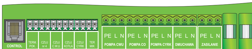
Rys. 3a Widok przyłączy regulatora
